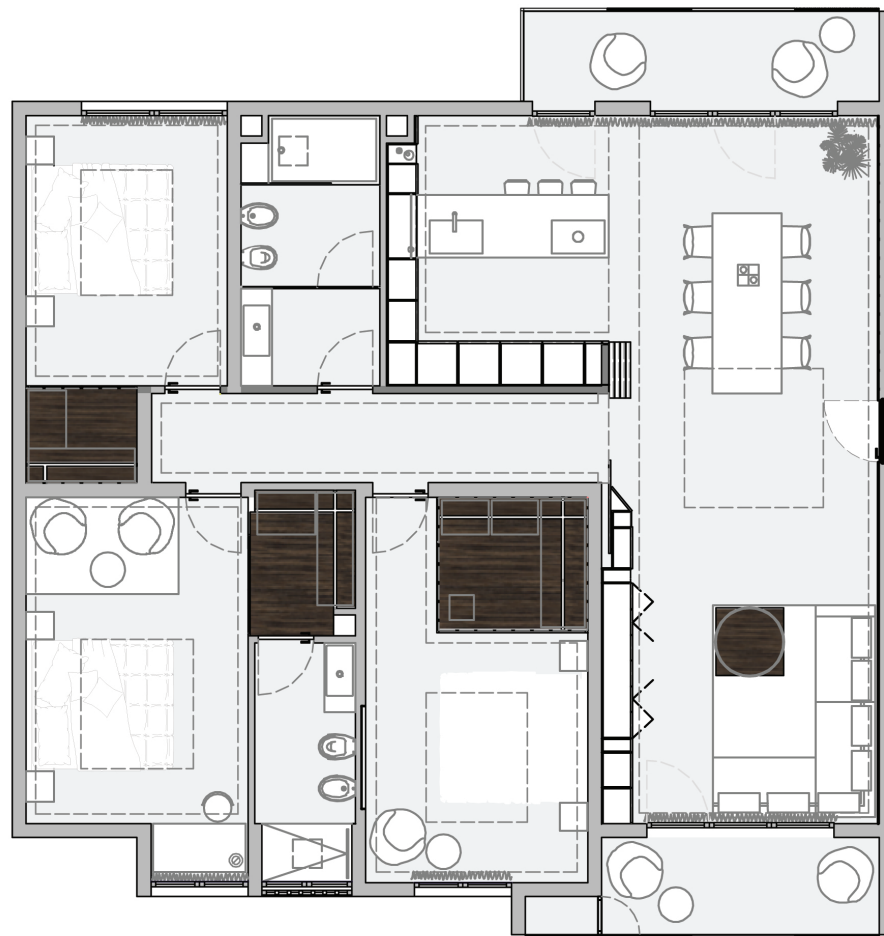
PIANTA PANNELLI APERTI
