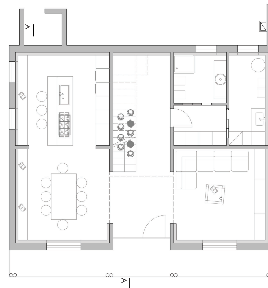
PIANTA APPARTAMENTO PIANO TERRA
